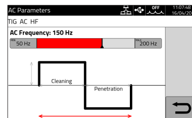
Regolazione rapida dei parametri della frequenza AC (solo per TIG AC-DC) Quick adjustment of AC frequency parameters (only for AC-DC TIG)
